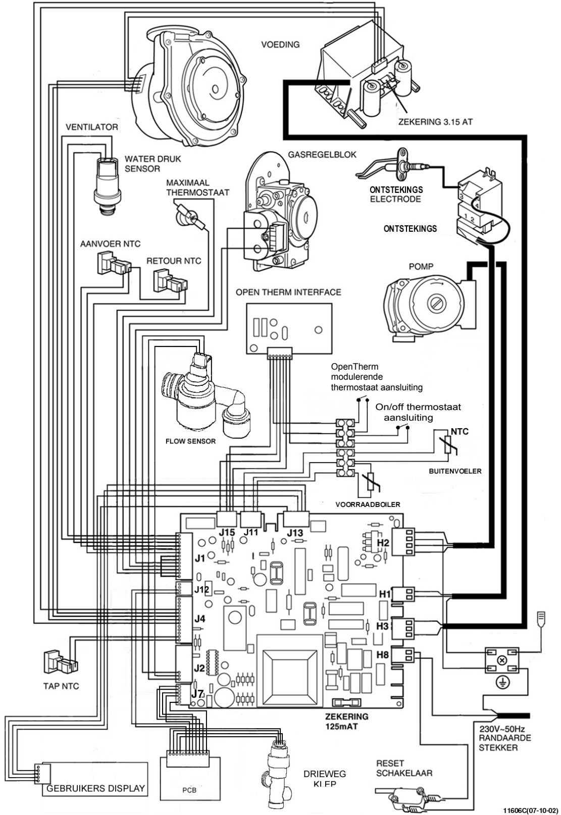
Figuur 16. Elektrisch schema
