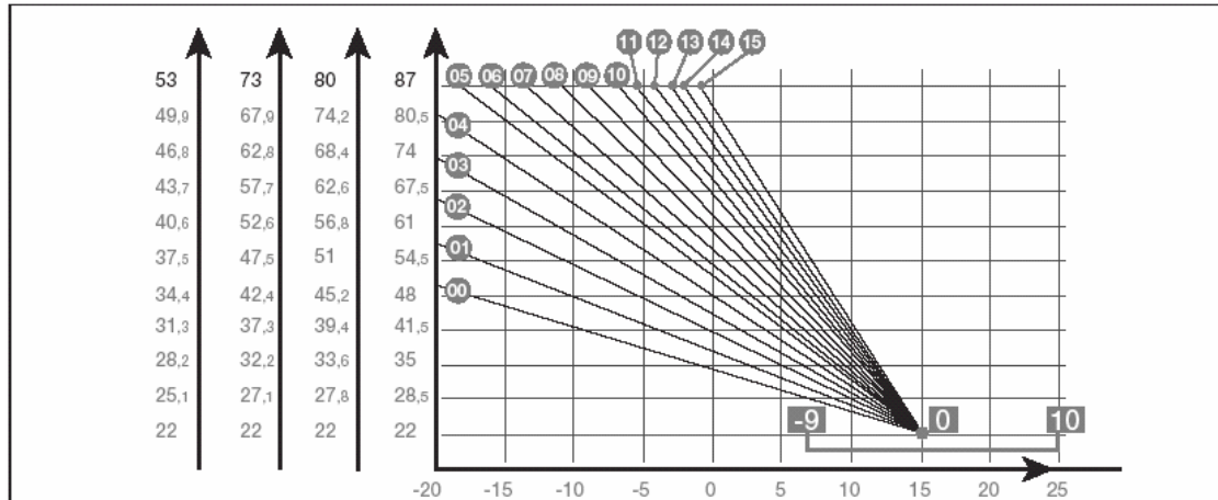
Figuur 13 Voorbeelden stooklijnstellingen
