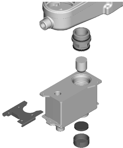
Figuur 9. Plaats bypass (kortsluitleiding)
