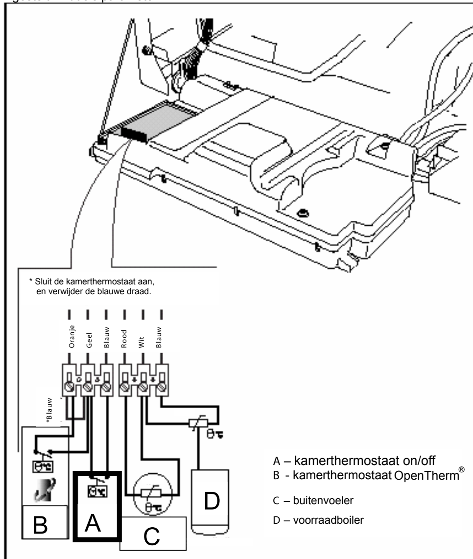
Figuur 12 Aansluitingen kamerthermostaat op 6-polige kroonsteen
